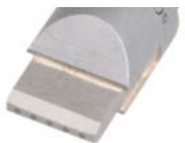
Diamant rhomboïde 5 x 0,6 x 0,6 mm, Surface d'appui 1,80 mm 2 , r = 0,40 mm
