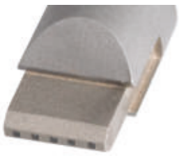
Rhomboid Diamant 6 x 0,5 x 0,5 mm RC, Gesamt-Tragfläche 1,5 mm 2 , r = 0,30 mm
