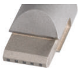
Diamant carré 5 x 0,7 x 0,7 mm, Surface d'appui 2,45 mm 2 , r = 0,42 mm
