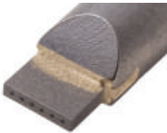
Rhomboid Diamant 6 x 0,5 x 0,5 mm RC, Gesamt-Tragfläche 1,5 mm 2 , r = 0,30 mm
