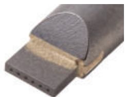
Diamant rhomboïde 6 x 0,5 x 0,5 mm RC, Surface d'appui 1,5 mm 2 , r = 0,30 mm
