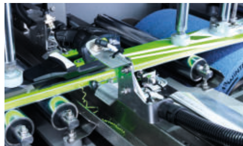
Trimcut-Automatisierte Seitenwangenvorbehandlung
