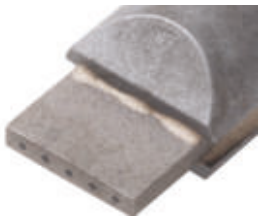
Rhomboid-Diamant 5 x 0,5 x 0,5 mm RC, Gesamt-Tragfläche 1,25 mm 2 , r = 0,33 mm
