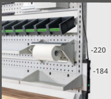
Porta rotolo di carta triplo Multipresa Schuko da 16 A / Papierrollenhalter 3-fach Schuko-Steckdosenleiste 16A
