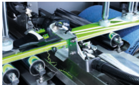
Trimcut-Automatisierte Seitenwangenvorbehandlung
